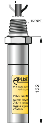
SGM type IP68
